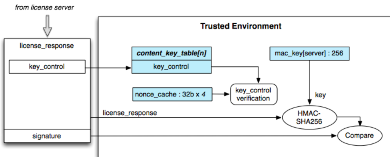
OEMCrypto_LoadKeys()
