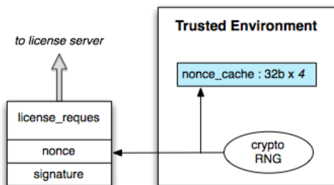
OEMCrypto_GenerateNonce()
