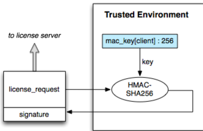
OEMCrypto_GenerateSignature()
