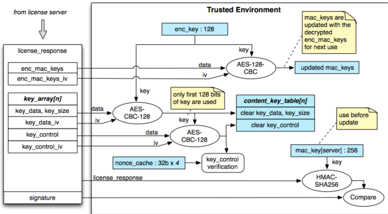
OEMCrypto_LoadKeys()
