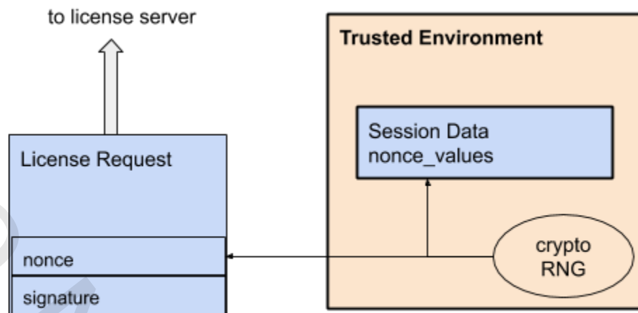
OEMCrypto_GenerateNonce
